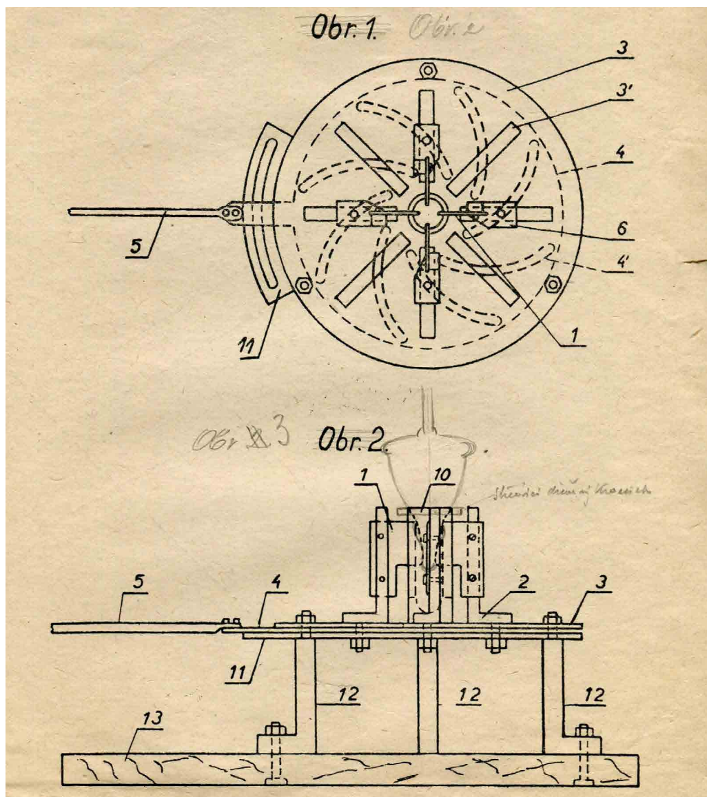
Obr. 3: Náčrt zařízení na tvarování stopek kalíšků – příloha patentního spisu č. 83405 s Tylčerovou kresbou, Písemná pozůstalost E. Tylčera.
